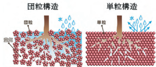
図 土壌の単粒構造と団粒構造
